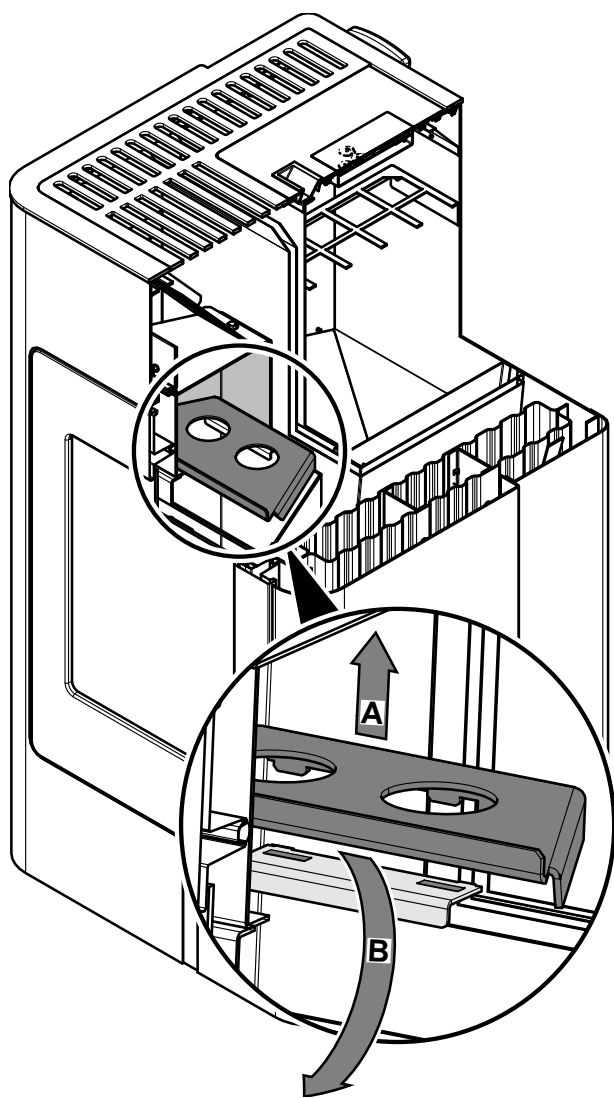
Obrázok 2: Demontáž obloženia ťahu
