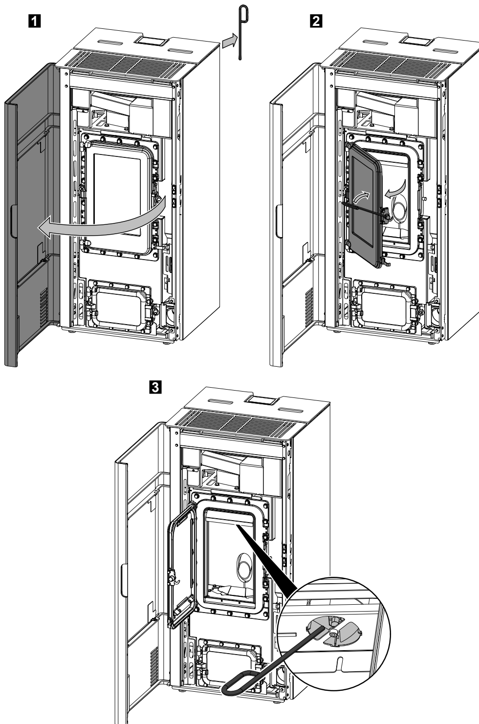
Obrázok 5: Čistenie deflektora
