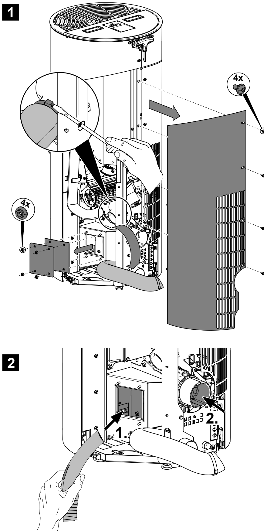
Obrázok 4: Demontáž bočnej steny
