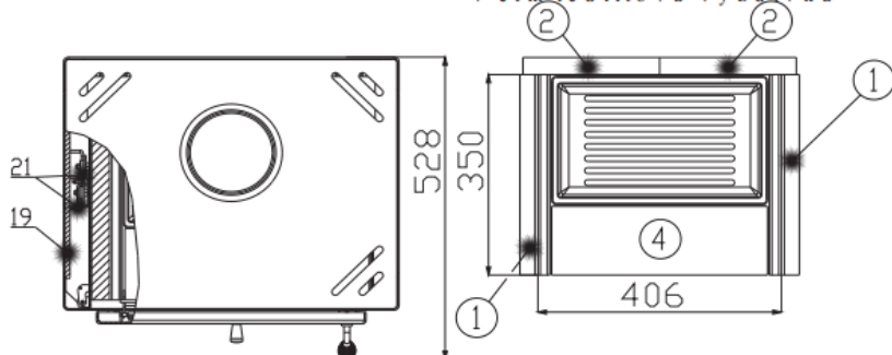
Vermiculitová vyzdívka
