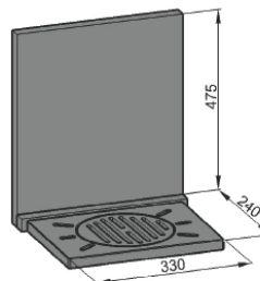
Informatívny rozměr topeniště
